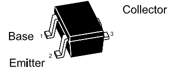
SOT-323
